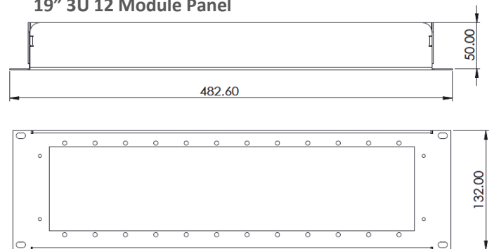
19" 3U 12 Module Panel
