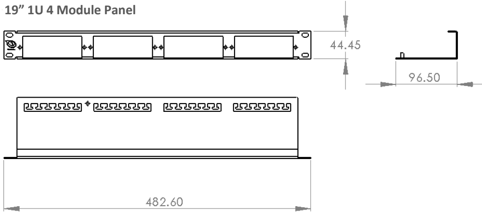
5 Port SIJ Faceplate
